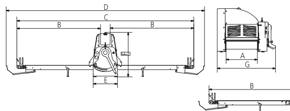
SF600-85/100/120/140
