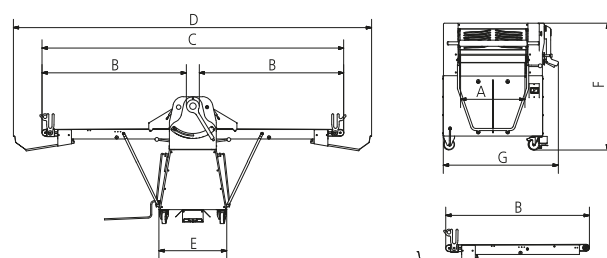
SF600-85/100/120/140
